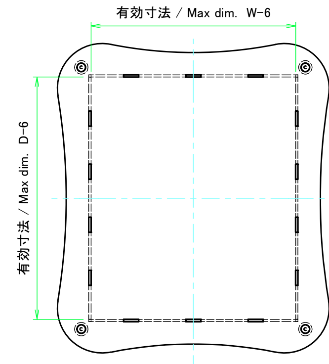
下カバー / Bottom cover
