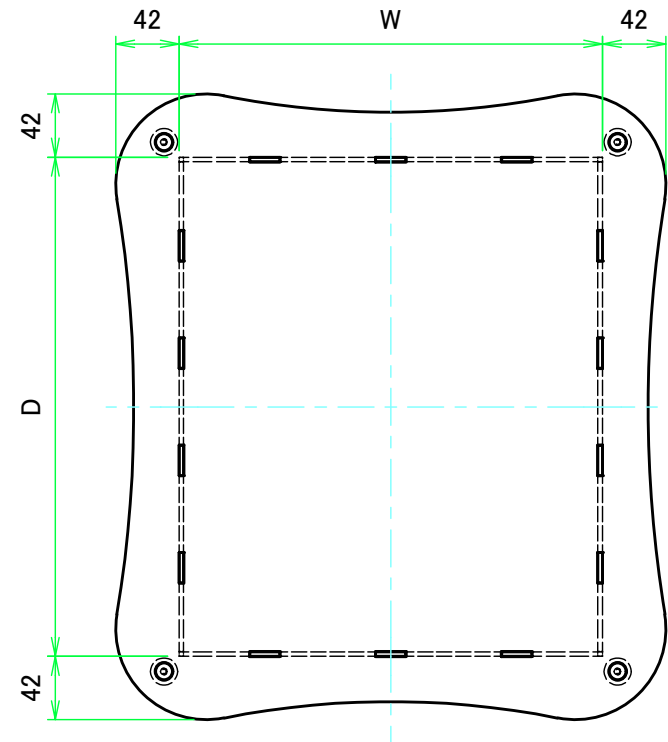
Wパネル1 / W panel 1
